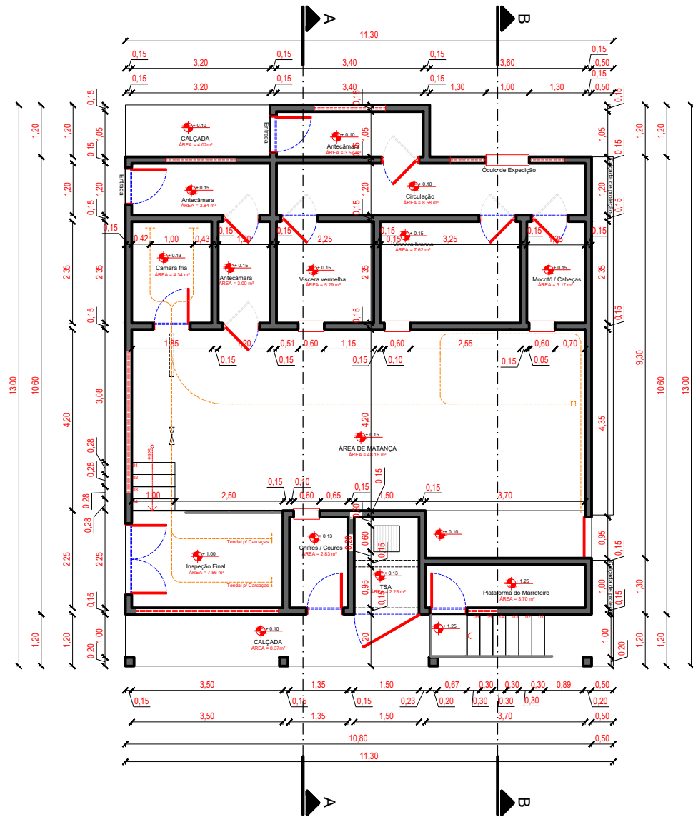
PLANTA BAIXA _ LAYOUT _ ÁREA DE MATANÇA ESCALA 1/125
